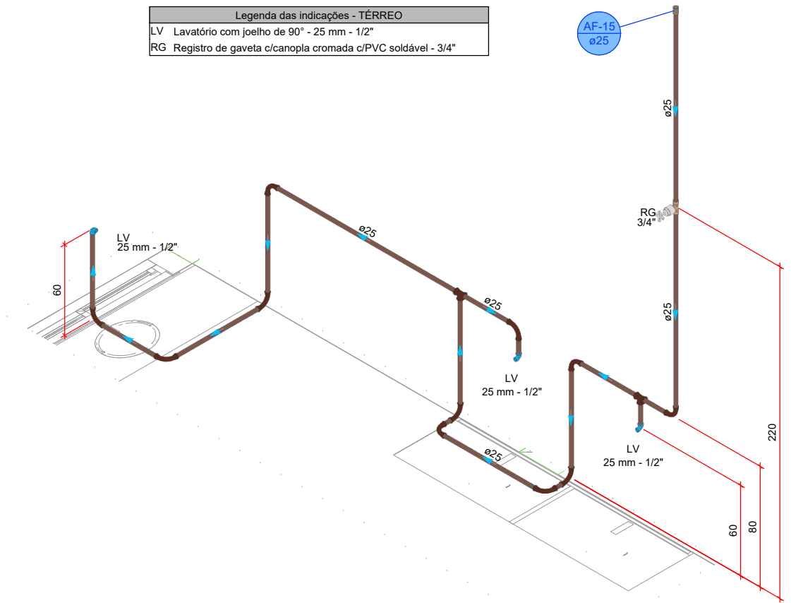
DETALHE H14 1:25
