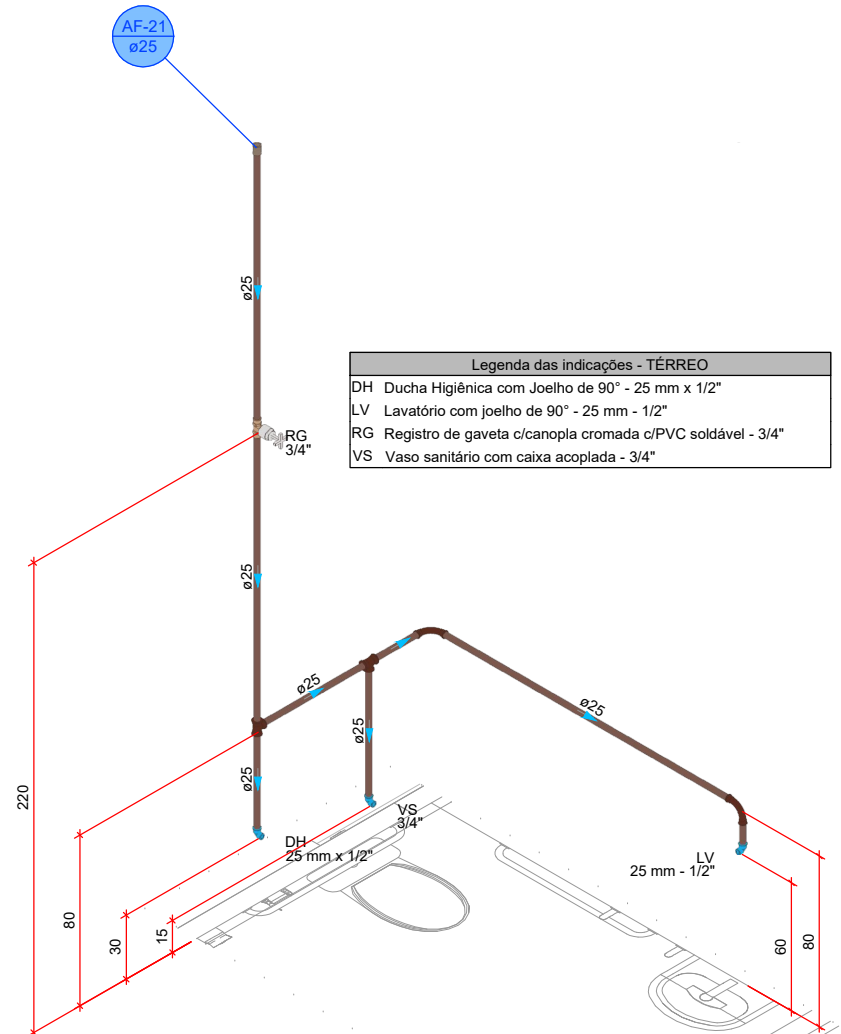
DETALHE HID-21 1:25
