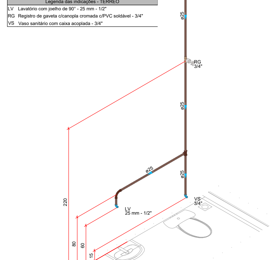
DETALHE HID-22 1:25
