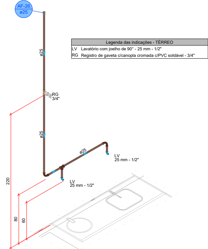
DETALHE HID-25 1:25
