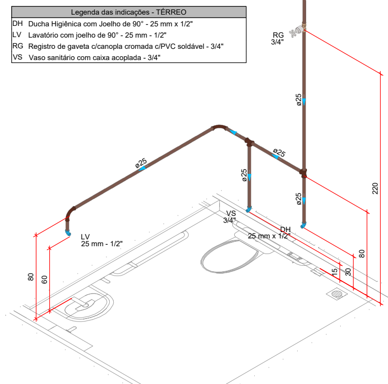
DETALHE HID-16 1:25
