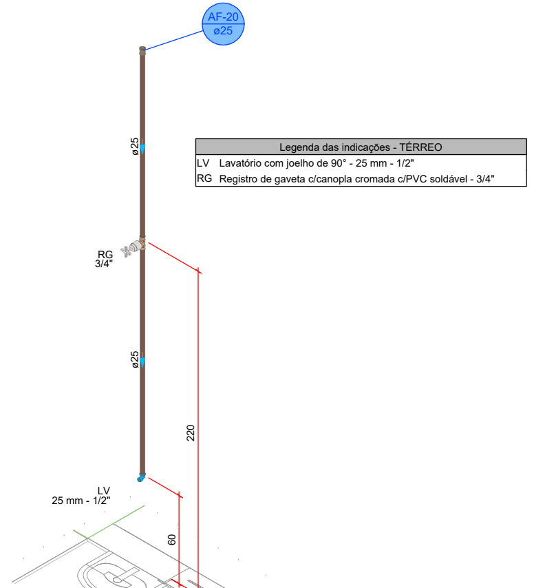
DETALHE HID-19 1:25
