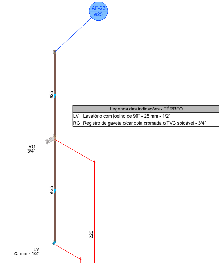
DETALHE HID-23 1:25
