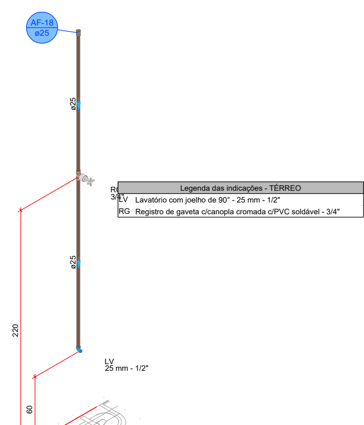
DETALHE HID-18 1:25
