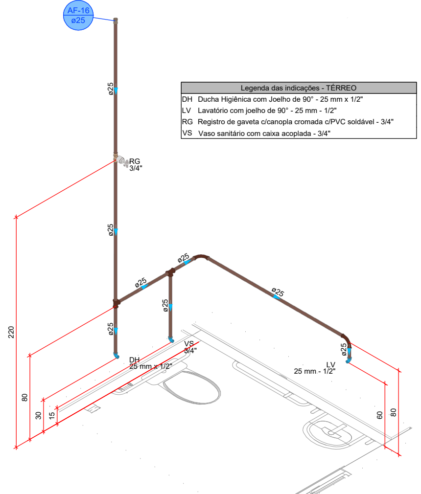
DETALHE HID-17 1:25
