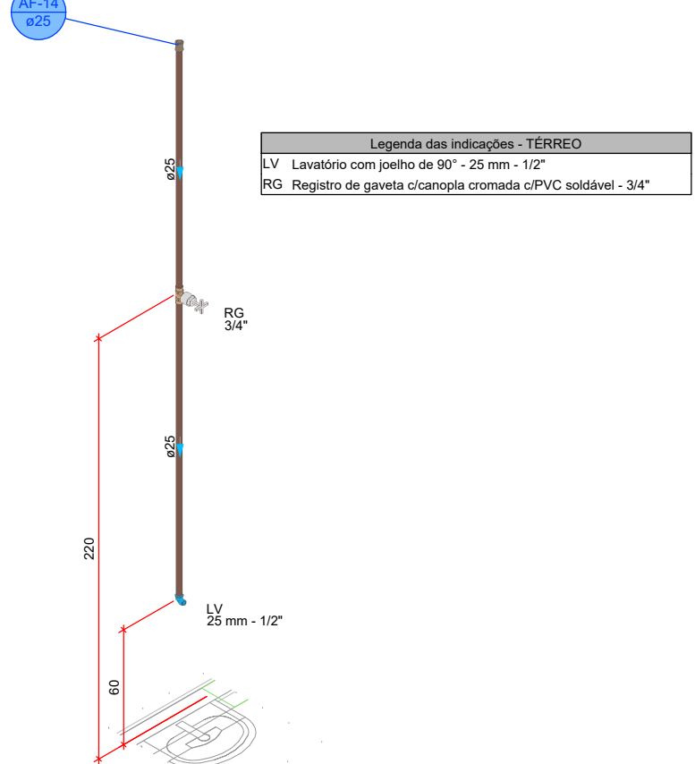
DETALHE HID-15 1:25
