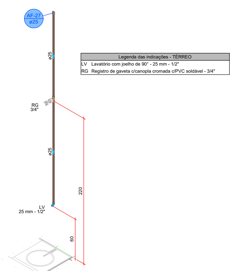
DETALHE HID-26 1:25
