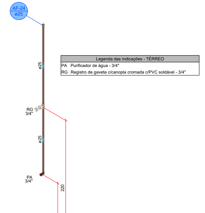
DETALHE HID-24 1:25
